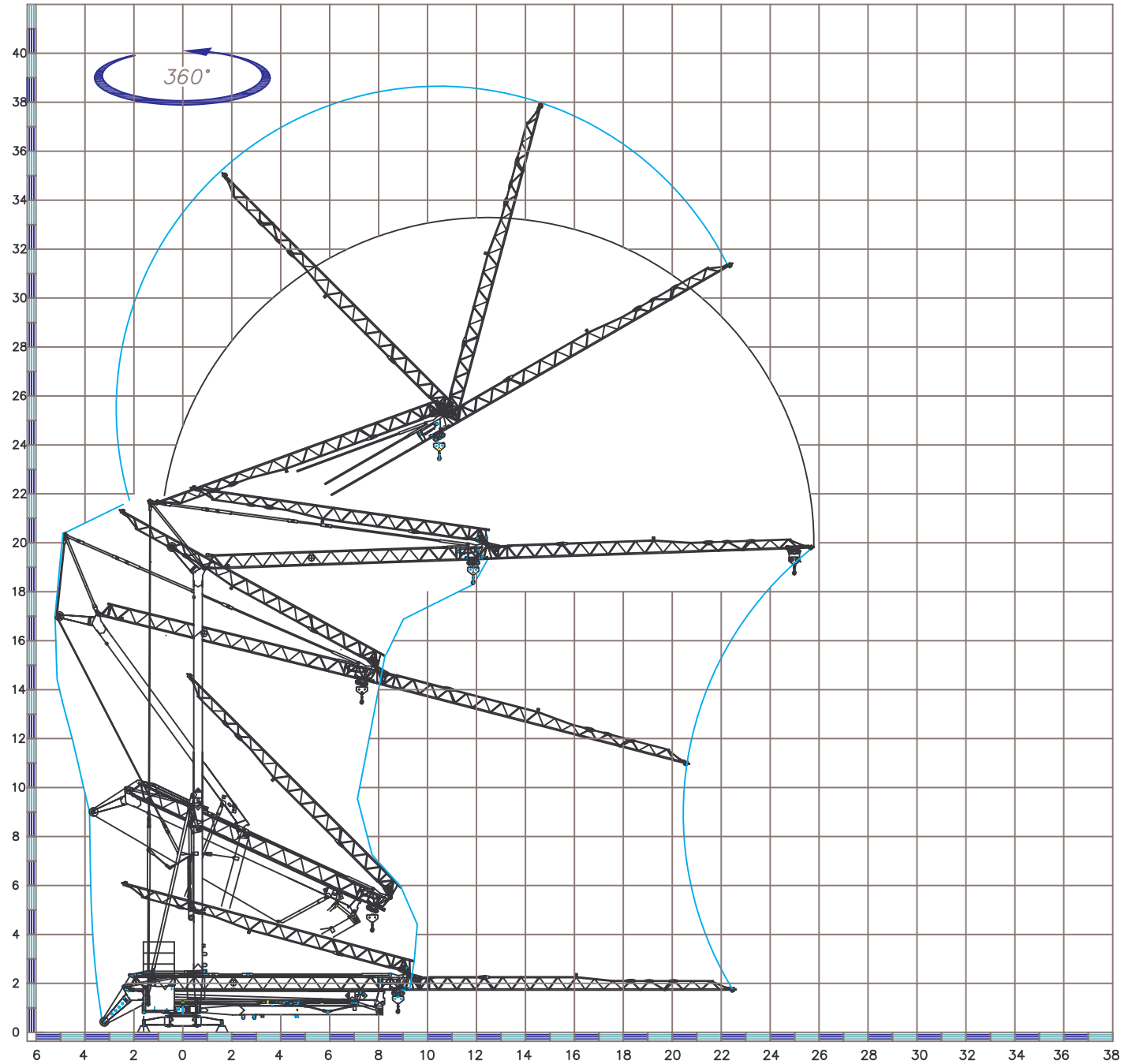
Sequenza di montaggio su 360°. Aufstellvorgang uber 360°. Déroulement de montage sur 360°. Erection procedure on 360°. Montaje sobre 360°.
