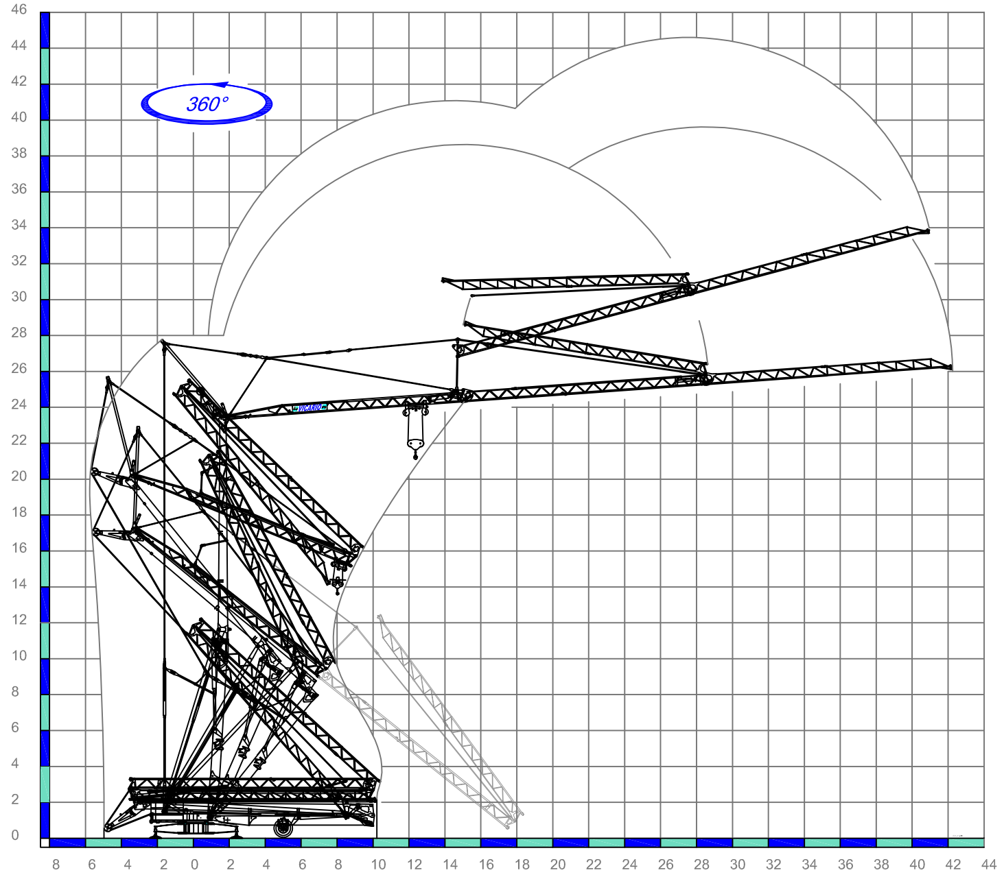
Sequenza di montaggio su 360°. Aufstellvorgang uber 360°. Dérulment de montage sur 360°. Erection procedure on 360°. Montaje sobre 360°.
